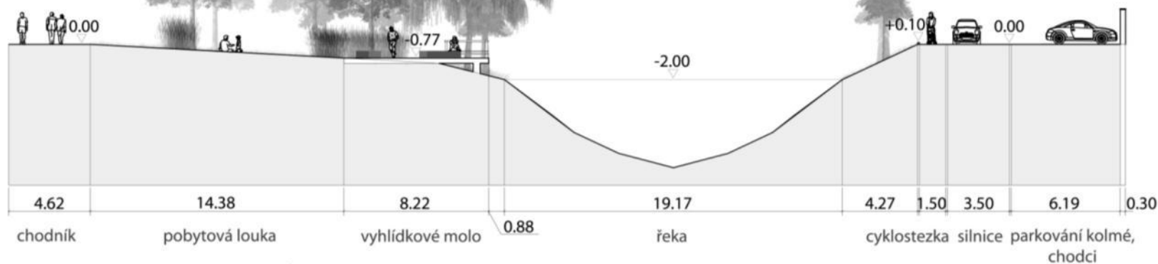
Řez BB'
