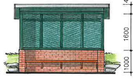
POHLED ČELNÍ
