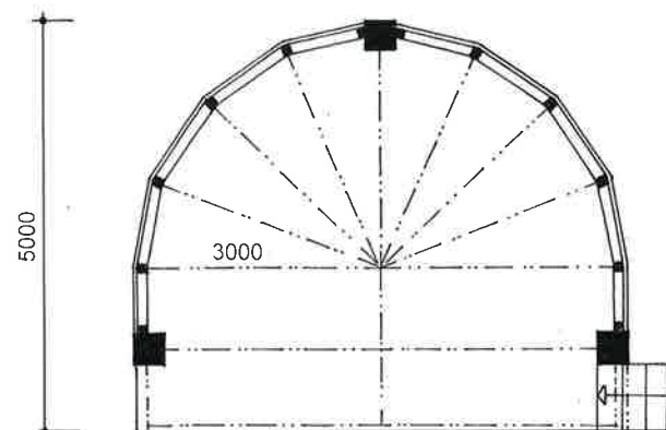
PŮDORYS
