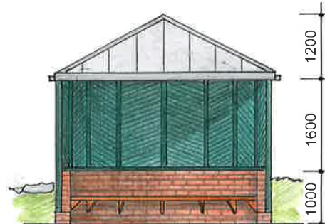
POHLED ČELNÍ
