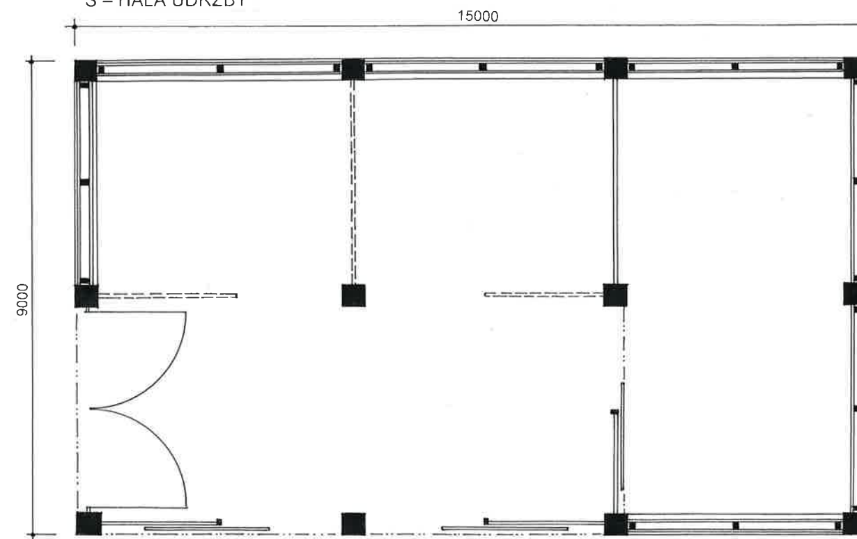
PŮDORYS
