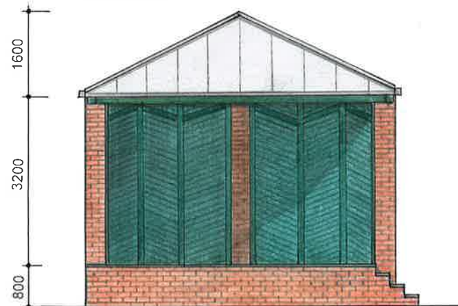
POHLED ČELNÍ
