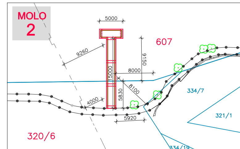
SITUACE MOLA 2 1:500
