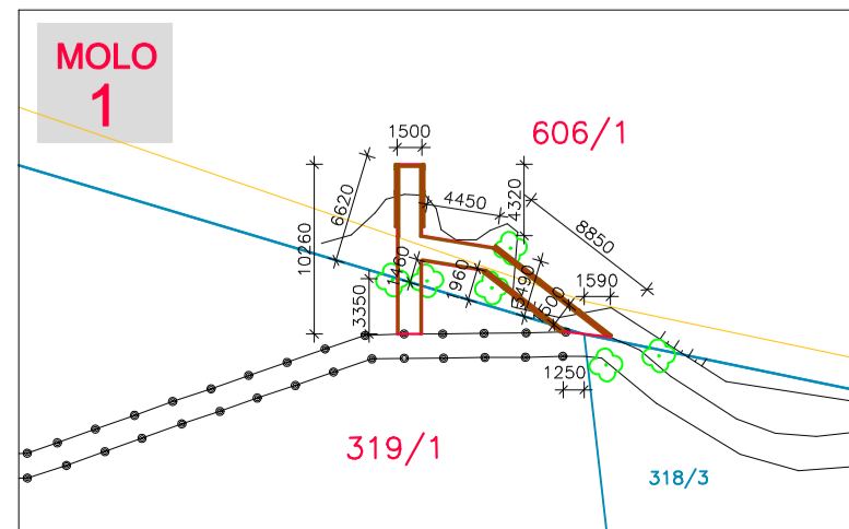
SITUACE MOLA 1 1:500
